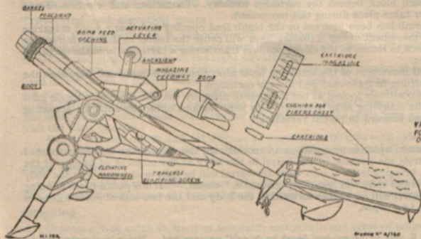
FIG. 18.—45 MM. MORTAR, MOD. 35—BRIXIA
